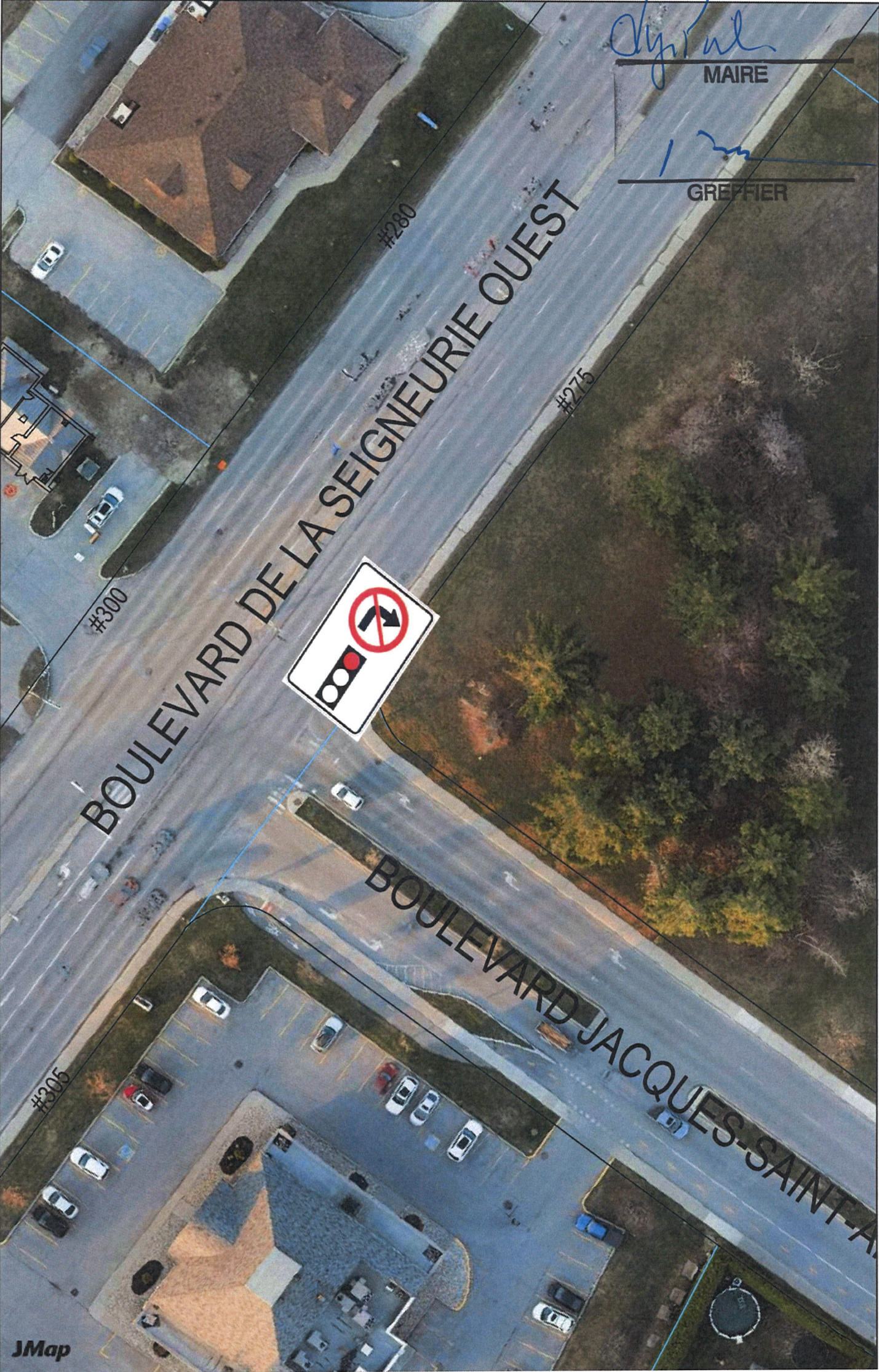
Croquis 2024-01 Ajout d'un panneau P-115-1 "Virage a droite interdit au feu rouge" à l'intersection "Boulevard de la Seigneurie Ouest / Boulevard Jacques-Saint-andré" 1:504
